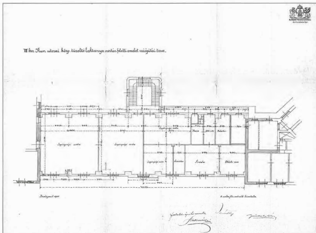
A szertár feletti emeletréépítés alaprajzi terve (Fővárosi Levéltár)
